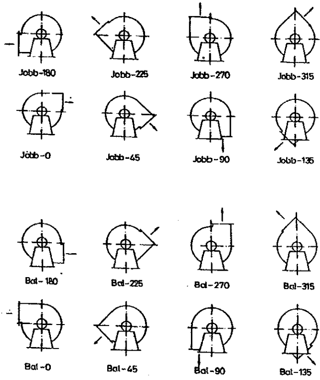
Házállás és forgásirány a motor felől nézve
